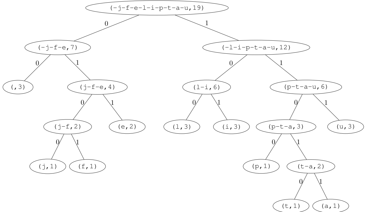
FIGURE 1 – arb-julie, un arbre de compression
